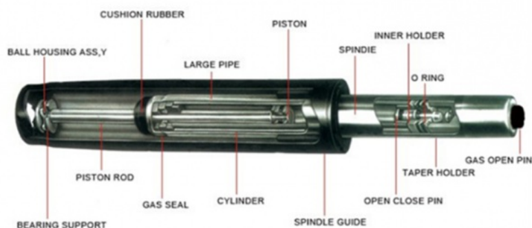
气压棒结构图 The Internal Structure
